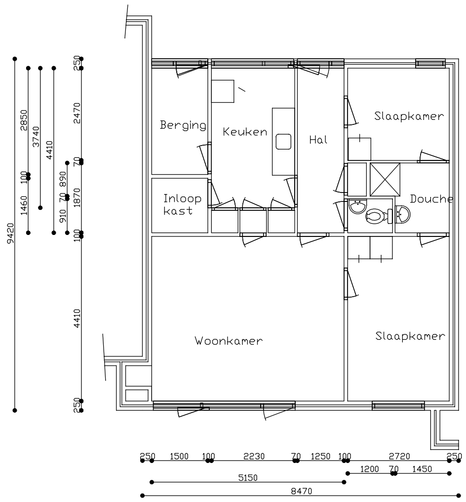
Begane grond
